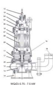
WQ(D) 0.75 - 7.5 kW
