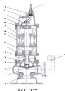
WQ 11 - 45 kW
