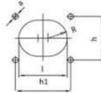
Kazan Bağlantı Flanşı Boiler Connection Flange фланец соединения котла
