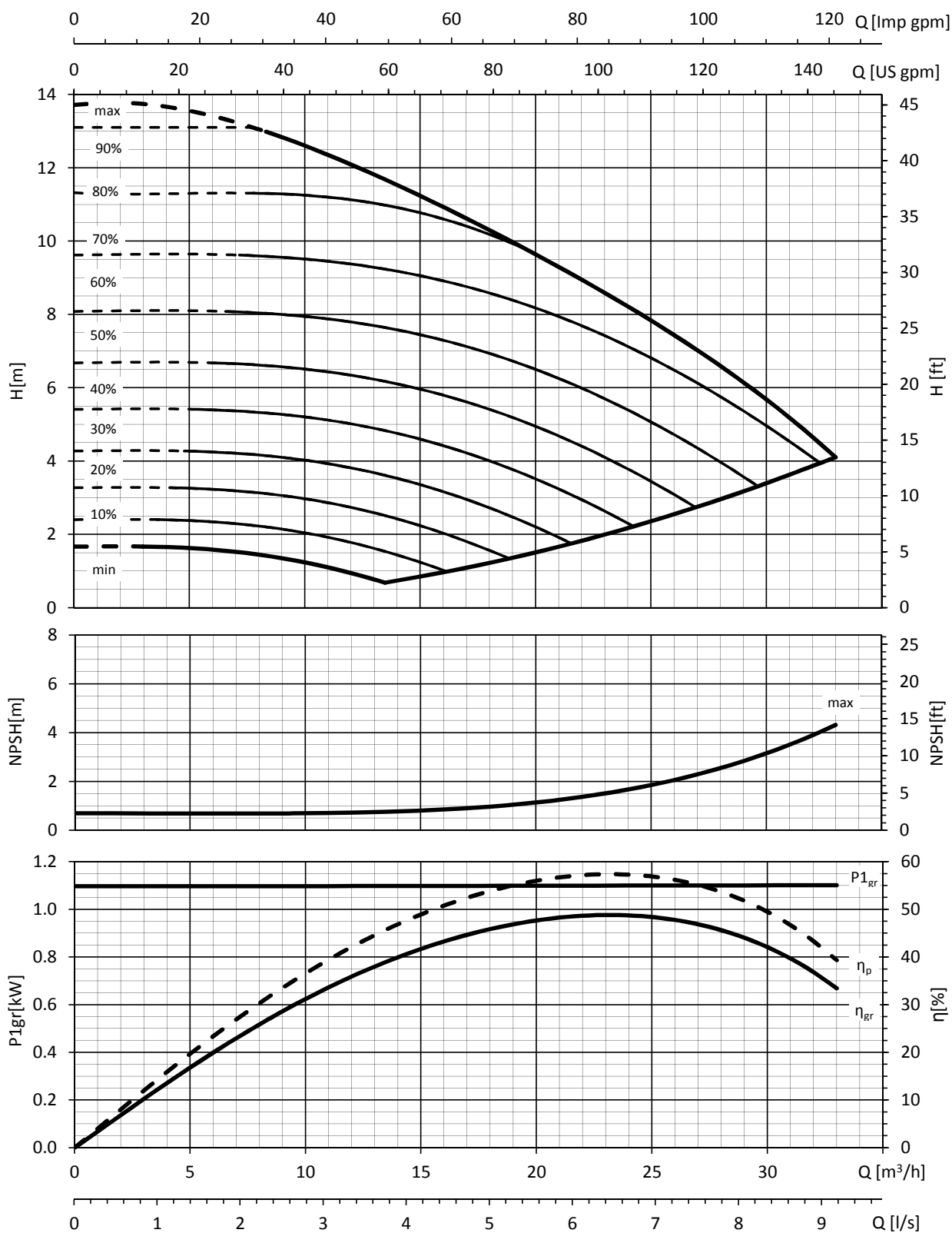
LNE..E 50-125/11/EP02
