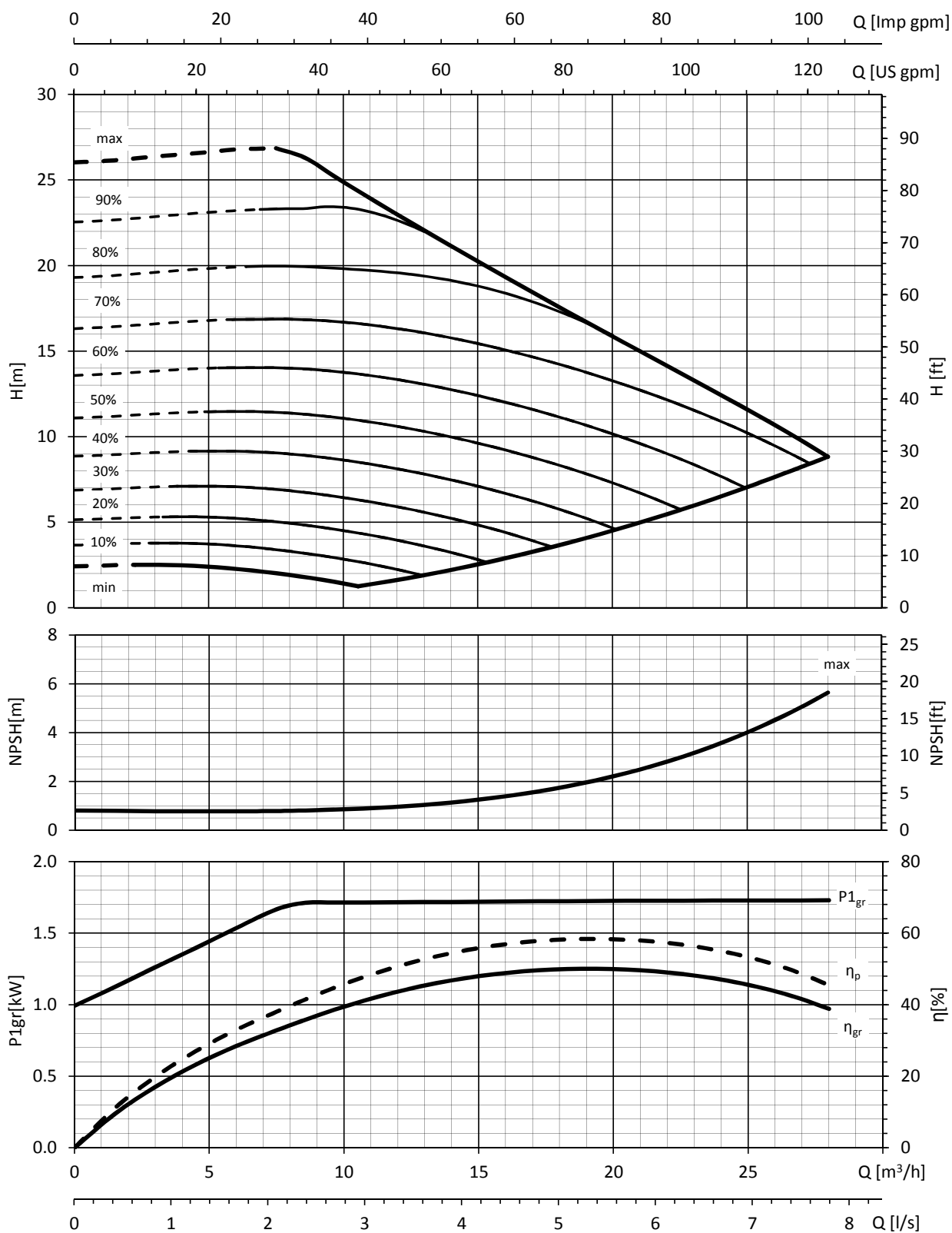
LNE..E 40-125/15/EP02
