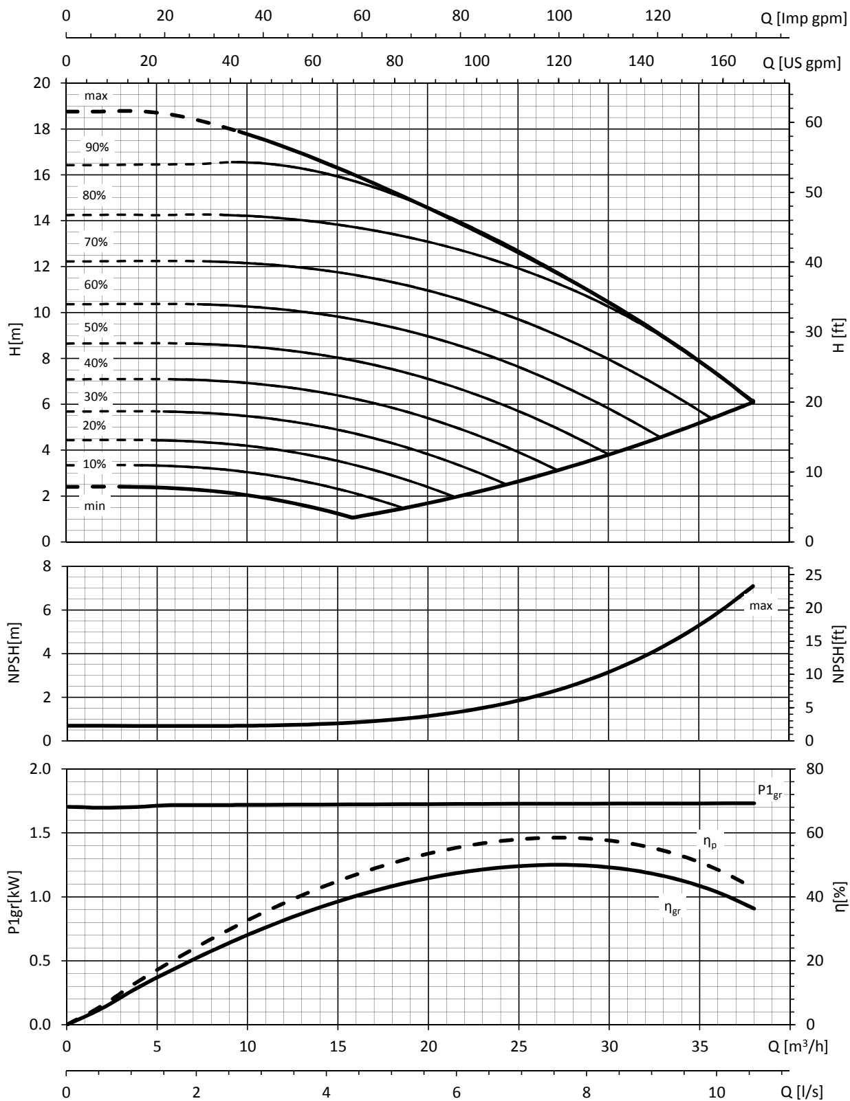
LNE..E 50-125/15/EP02
