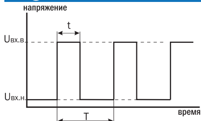
Рис.13 Характеристики ШИМ-сигнала
