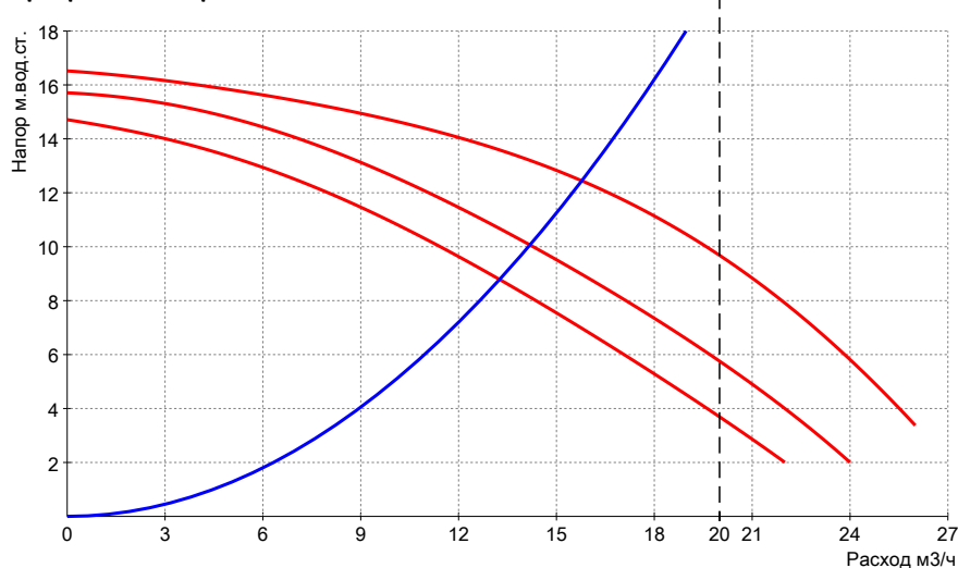
График подбора насоса:
