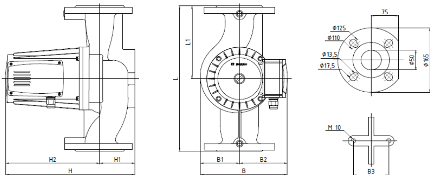
Чертеж насоса:
