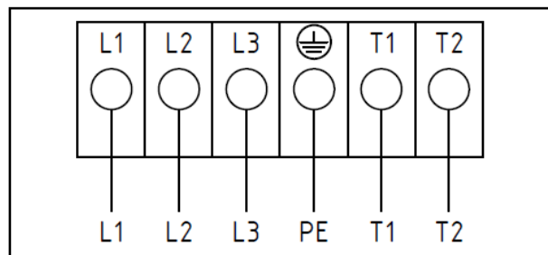
Электрическая схема насоса:
