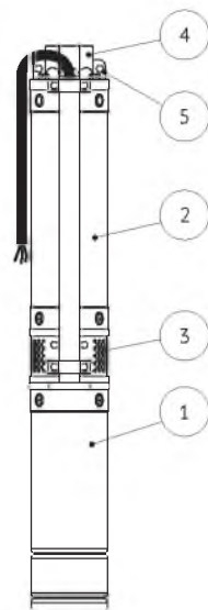
Рисунок 1 - Устройство агрегата
