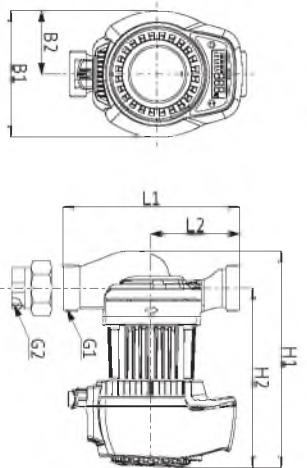
Рис. 2. Модель LPA **80
