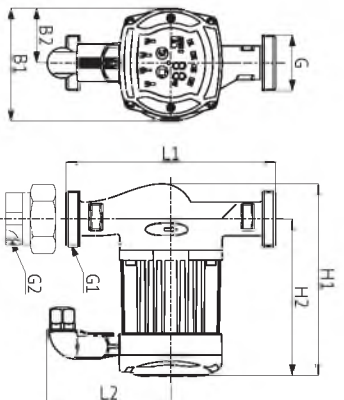
Рис. 1. Модели LPA **40, LPA **60
