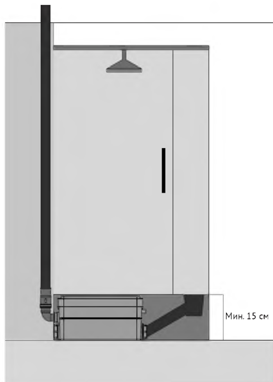
Рисунок 5 – Установка КНС под душевым поддоном
