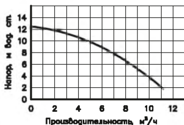
Диаграмма характеристик насоса WCP 50-12F
