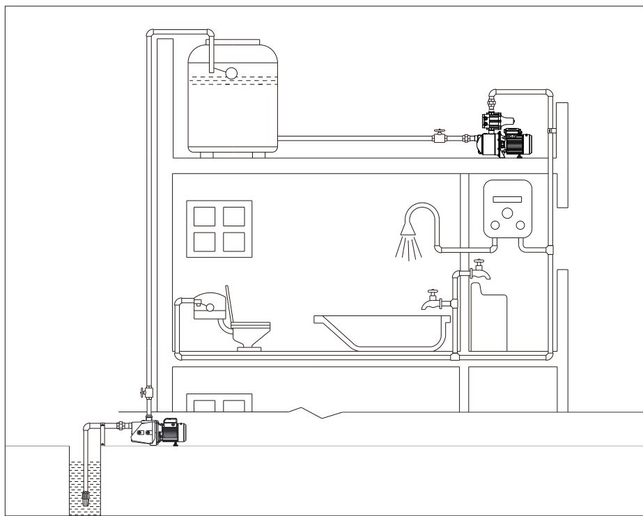
Подача воды из колодца
