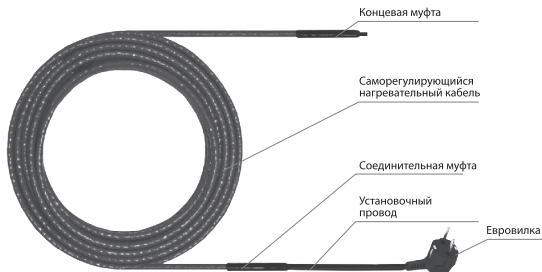
Рис. 1 - Конструкция секции нагревательной кабельной Freezstop Inside Dachha
