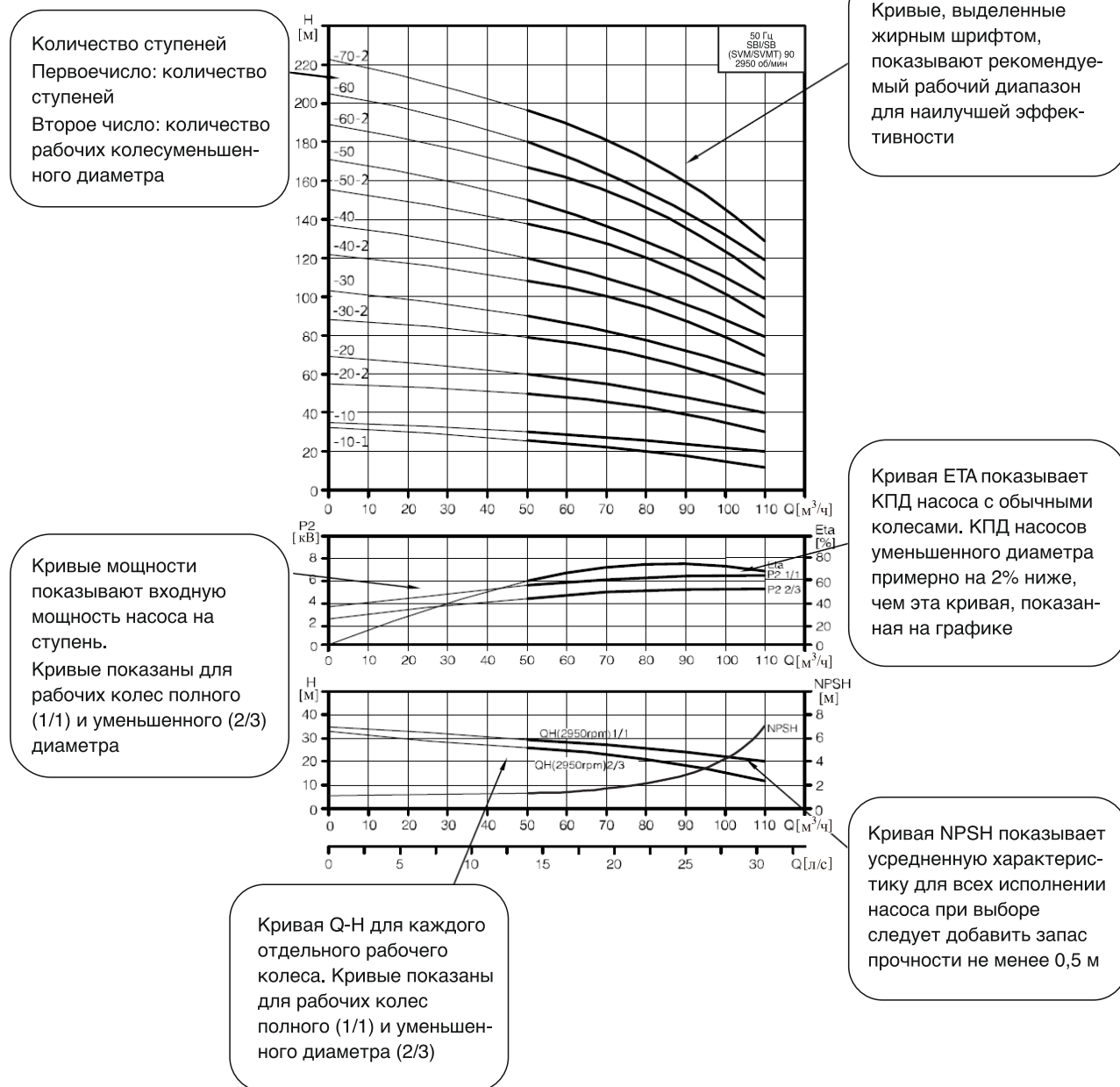
Кривая производительности
