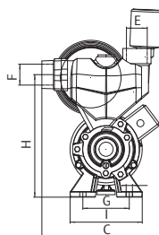
Габаритные и присоединительные размеры AUPS 550, AUPS 750, AUPS 1100
