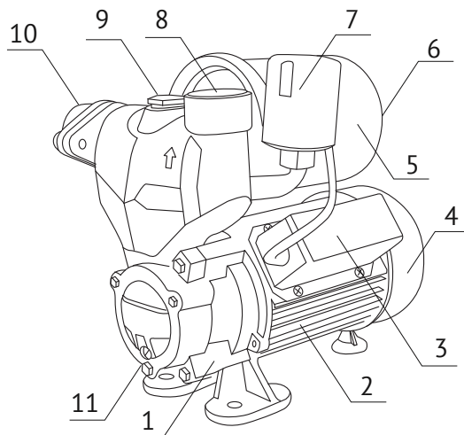
Рисунок 1 - Общий вид
