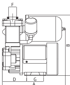
Габаритные и присоединительные размеры AUPS 126
