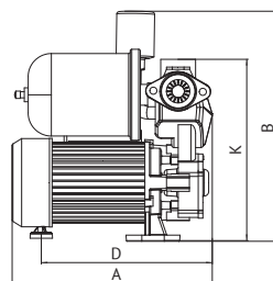
Габаритные и присоединительные размеры AUPS 550, AUPS 750, AUPS 1100
