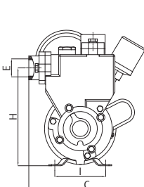
Габаритные и присоединительные размеры AUPS 126
