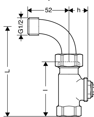
Рис. 5. Прямой с изогнутым патрубком
