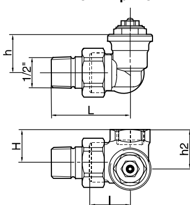
Рис. 4. Угловой торцевой
