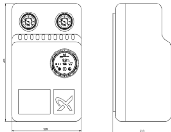
Рис. 2. Габаритные размеры
