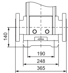
DIN FLANGE(LVR)/F
