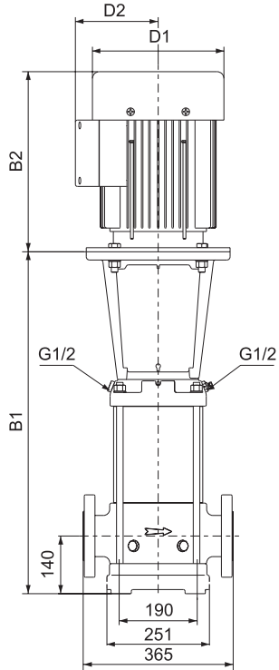
DIN FLANGE(LVS)/F
