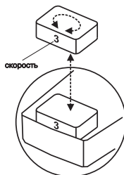
Рис.5. Переключение скорости трехфазного насоса.
