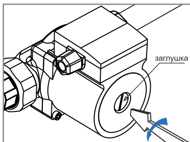
Рис.6. Удаление воздуха из корпуса насоса.
