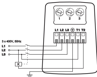
Рис.4. Схема подключения трехфазного насоса.
