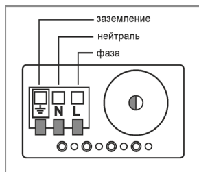
Рис.3. Схема подключения однофазного насоса.
