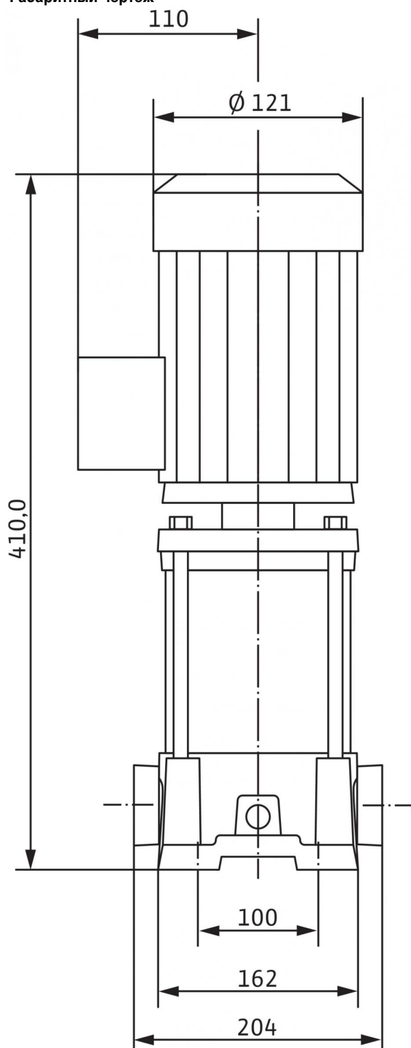
Габаритный чертеж
