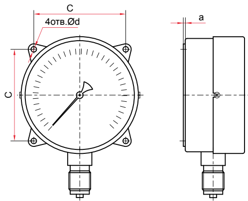
Исполнение с задним фланцем и радиальным присоединением (Ø100, 150 мм)
