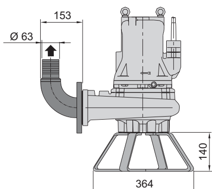
Модификация со стойкой и коленом 90°
