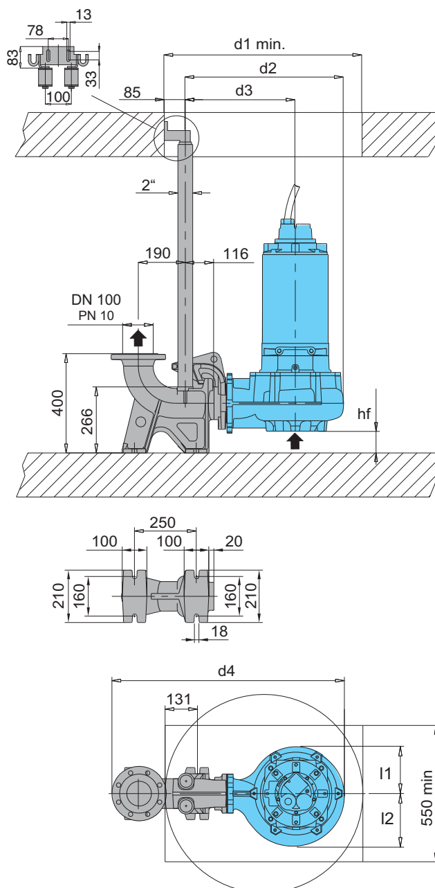
Модификация с соединительным желобом
