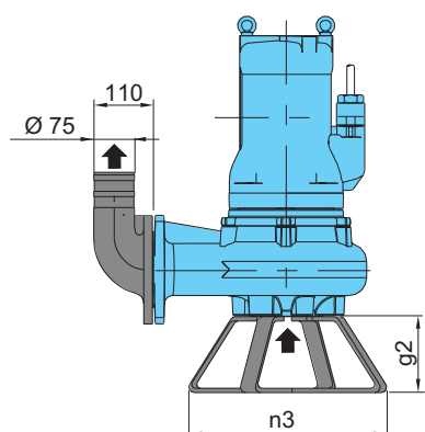
Модификация со стойкой и коленом 90°
