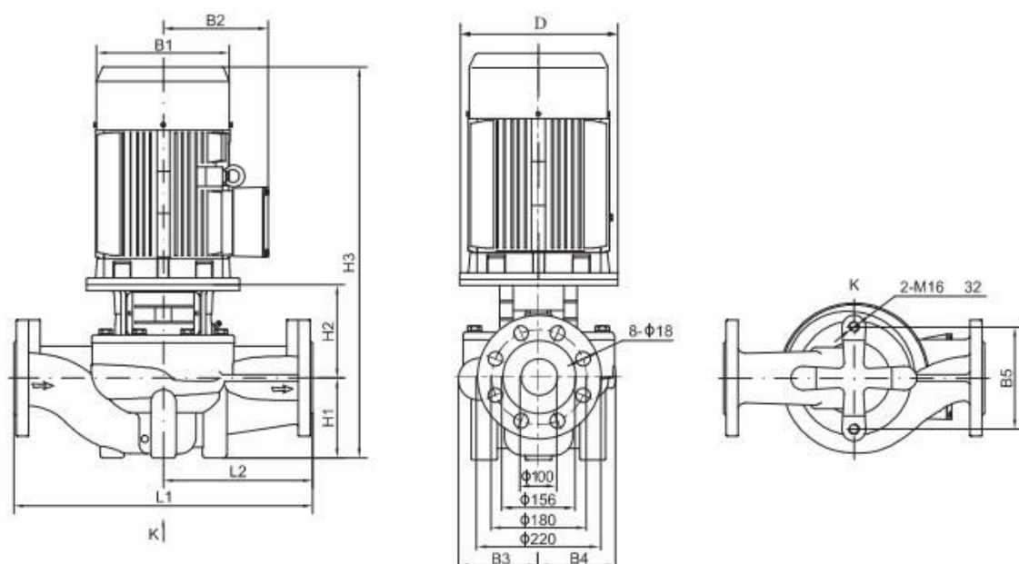
Установочные и габаритные параметры насосов серии DN100
