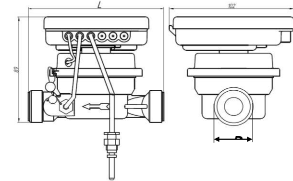
Приложение А ГАБАРИТНЫЙ ЧЕРТЕЖ И УСТАНОВОЧНЫЕ РАЗМЕРЫ
