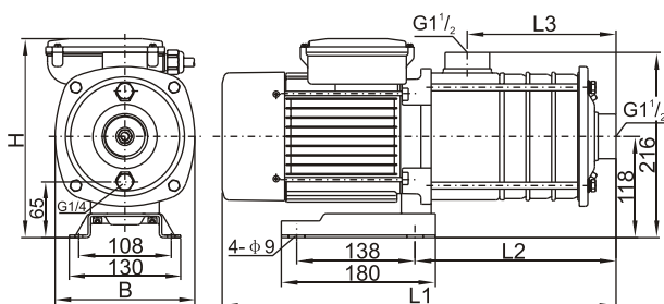
Габаритный чертеж
