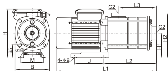
Габаритный чертёж
