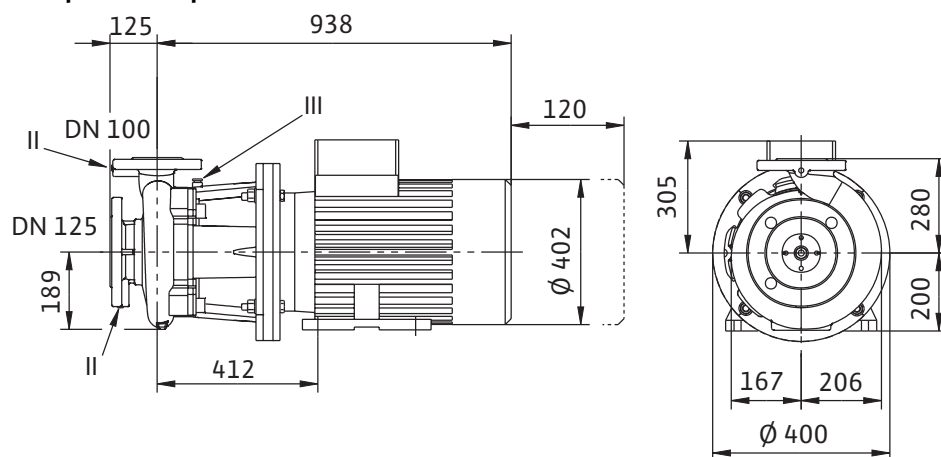
Габаритный чертеж
